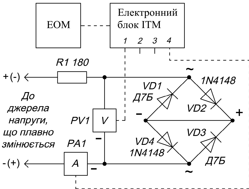
Рис. 9. Схема для отримання ВАХ діодного містка
